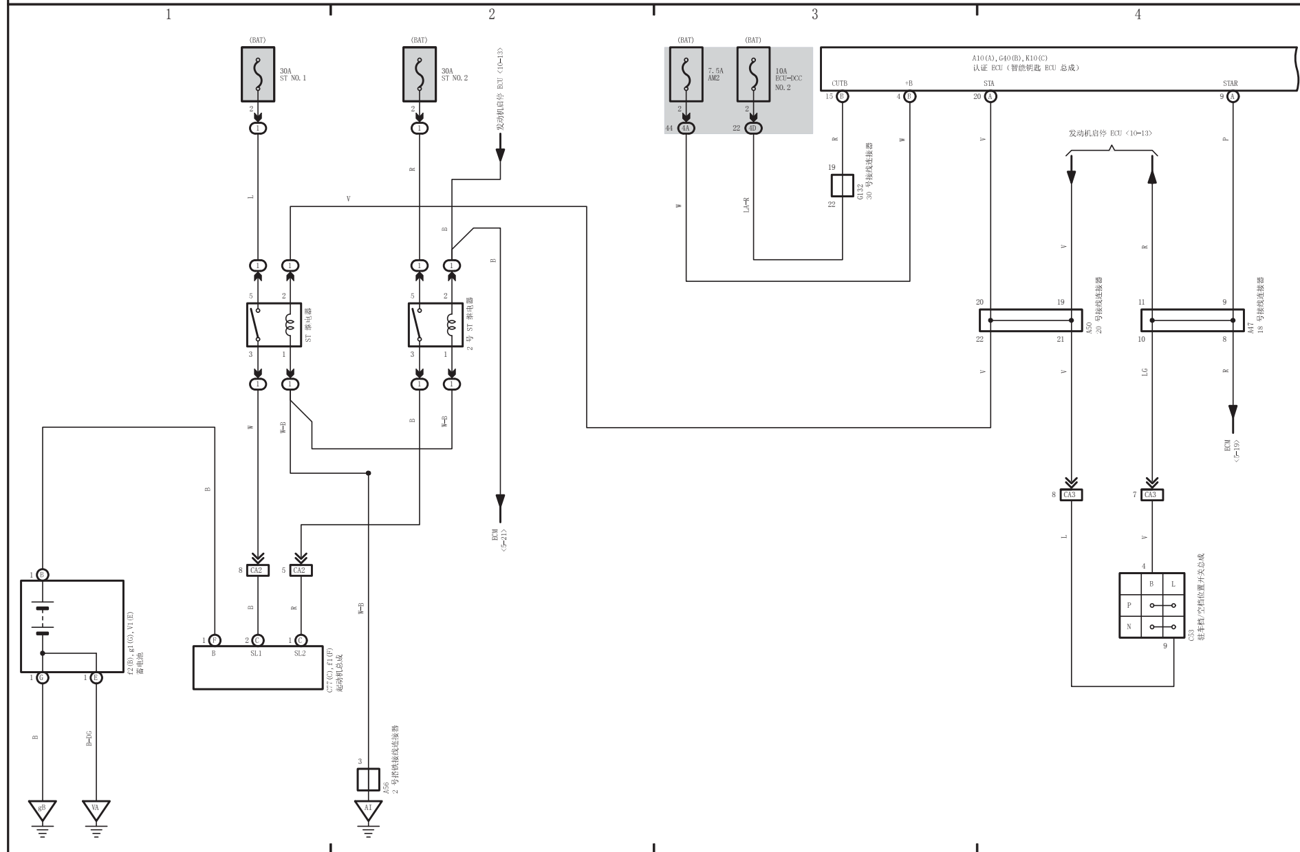
停机系统 (A25A-FKS)、起动 (A25A-FKS)、转向锁止 (A25A-FKS)、 智能上车和起动系统 (A25A-FKS)、遥控门锁控制 (A25A-FKS)
